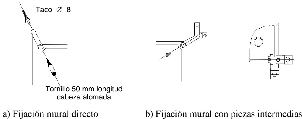
Figura 9.- Dispositivos de fijación de CGP
