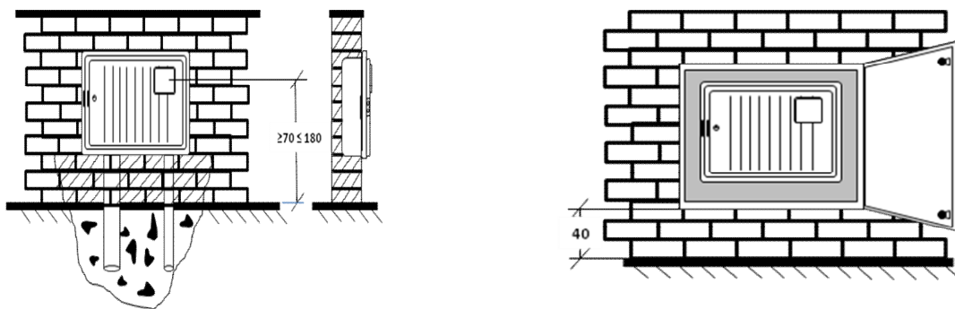
Figura 11.a) - Montaje CPM empotrada en valla Figura 11.b) - Montaje en nicho de pared
