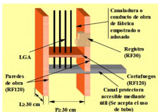
Figura 12.- Detalle de LGA
