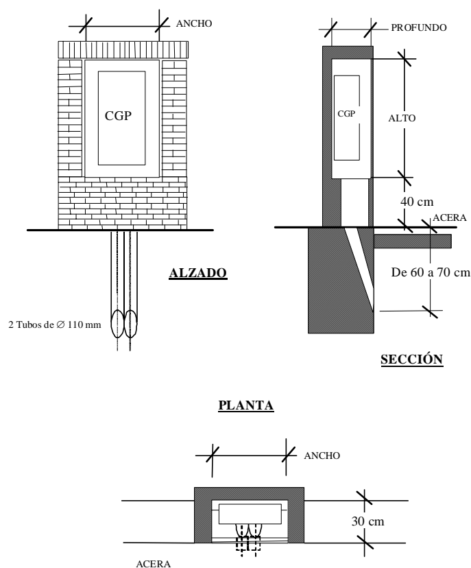
Figura 6.- Nicho para CGP
